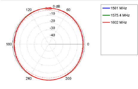
XY Plane: 1561-1602 MHz
