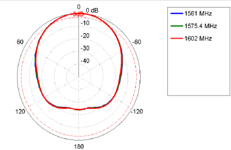
XZ Plane: 1561-1602 MHz
