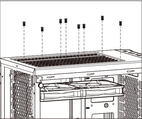
(7d) Install Top Fan x 2
