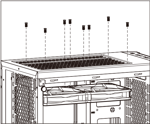
(7d) Install Top Fan x 2
