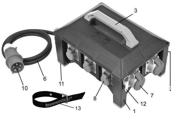
Abb. A, Bsp. Stromverteiler BSV 5 3/6 N560
